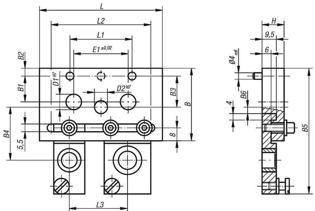
Bohrbuchsenträger-Platte
